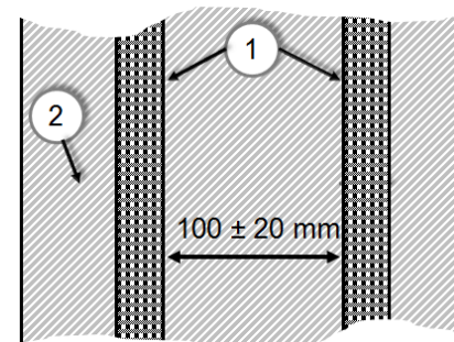
1 Armierungselemente 2 Wandung
